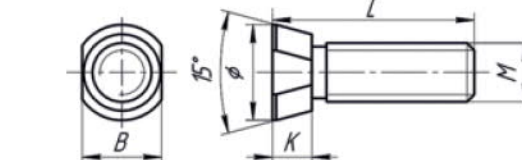
БОЛТ С 2-мя УСАМИ ISO 5713
