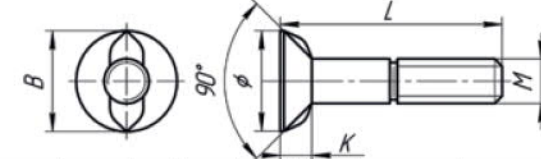
БОЛТ КОНУСНЫЙ С 2-мя ПЛОСКИМИ ГРАНЯМИ
