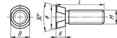
БОЛТ КОНУСНЫЙ С 1-ой ПЛОСКОЙ ГРАНЬЮ
