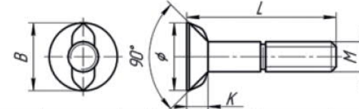
БОЛТ КОНУСНЫЙ С 2-мя ПЛОСКИМИ ГРАНЯМИ
